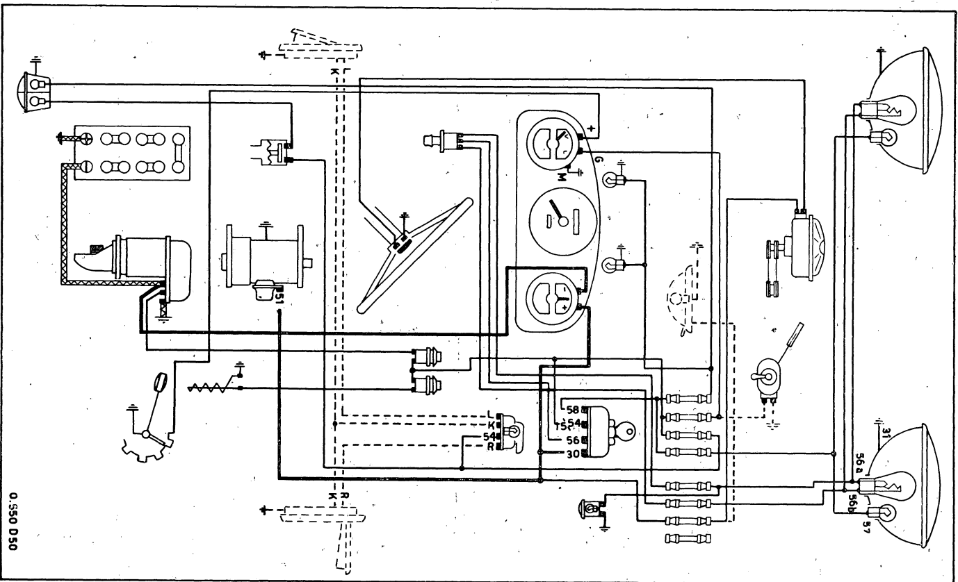
Schema elektrische installatie voor chassis met dieselmotor
