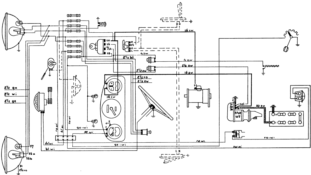
Schema elektrische installatie voor chassis met dieselmotor
