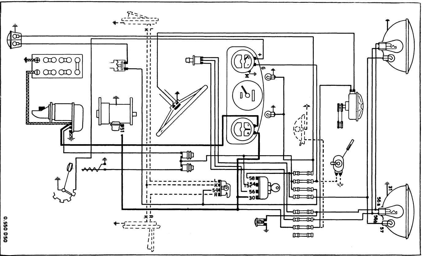
Schema elektrische installatie voor chassis met dieselmotor
