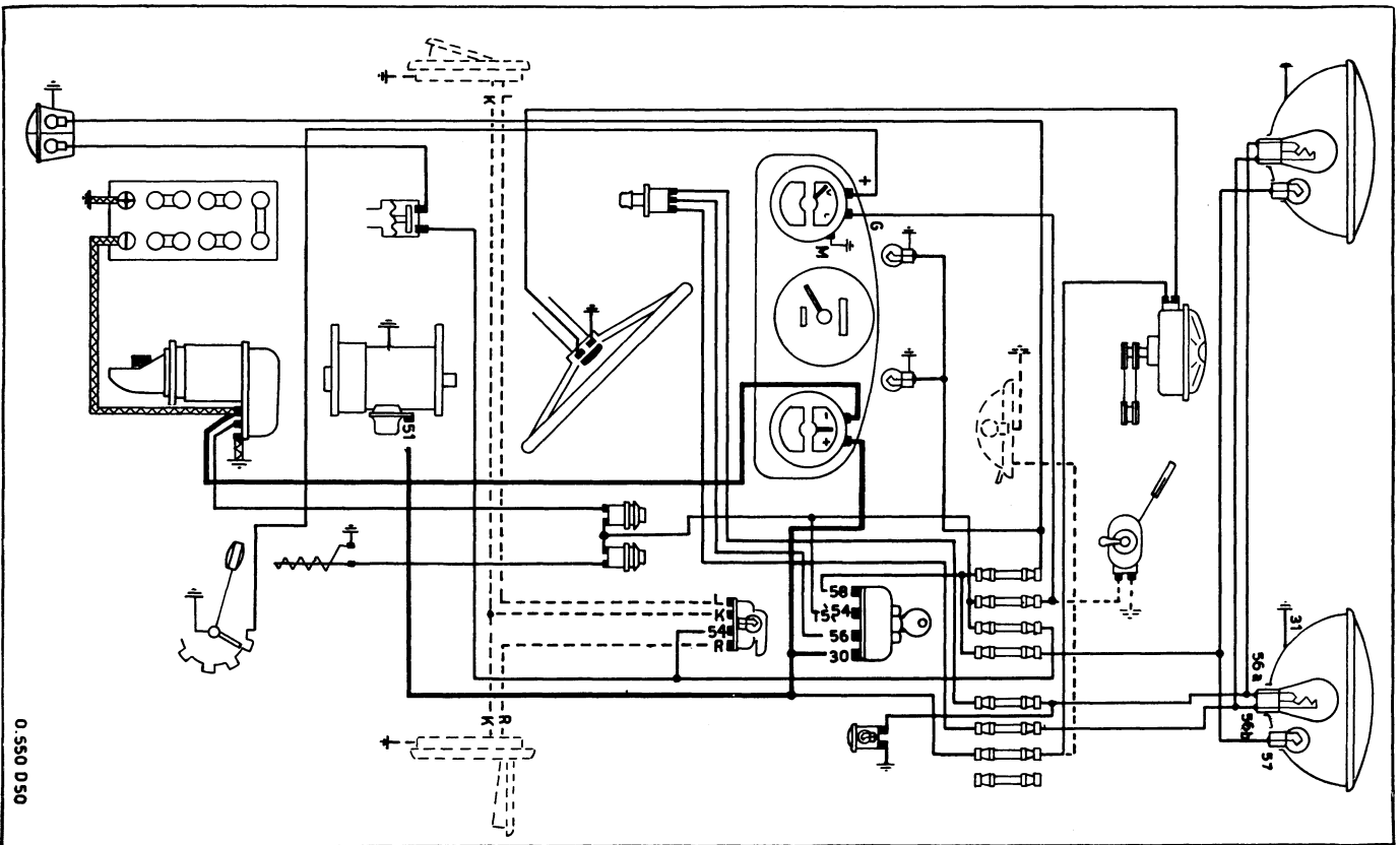
Schema elektrische installatie voor chassis 60P
