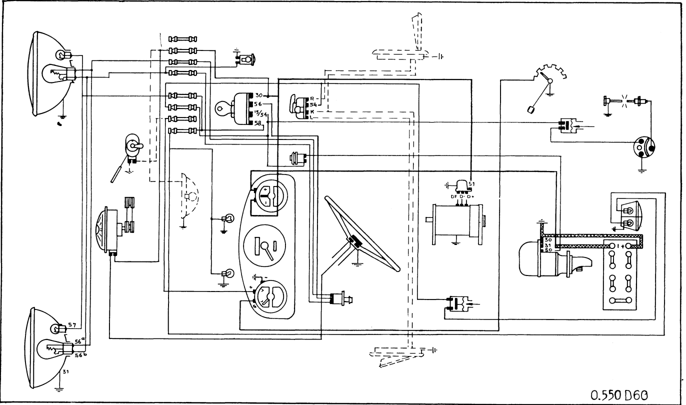
Schema elektrische installatie voor chassis 60 met dieselmotor (12 volts starter)
