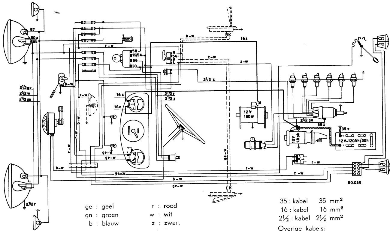
Schema elektrische installatie vrachtwagenchassis met benzinemotor
