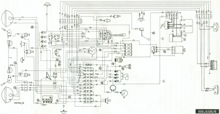
Afb. 30. Schema elektrische installatie.
