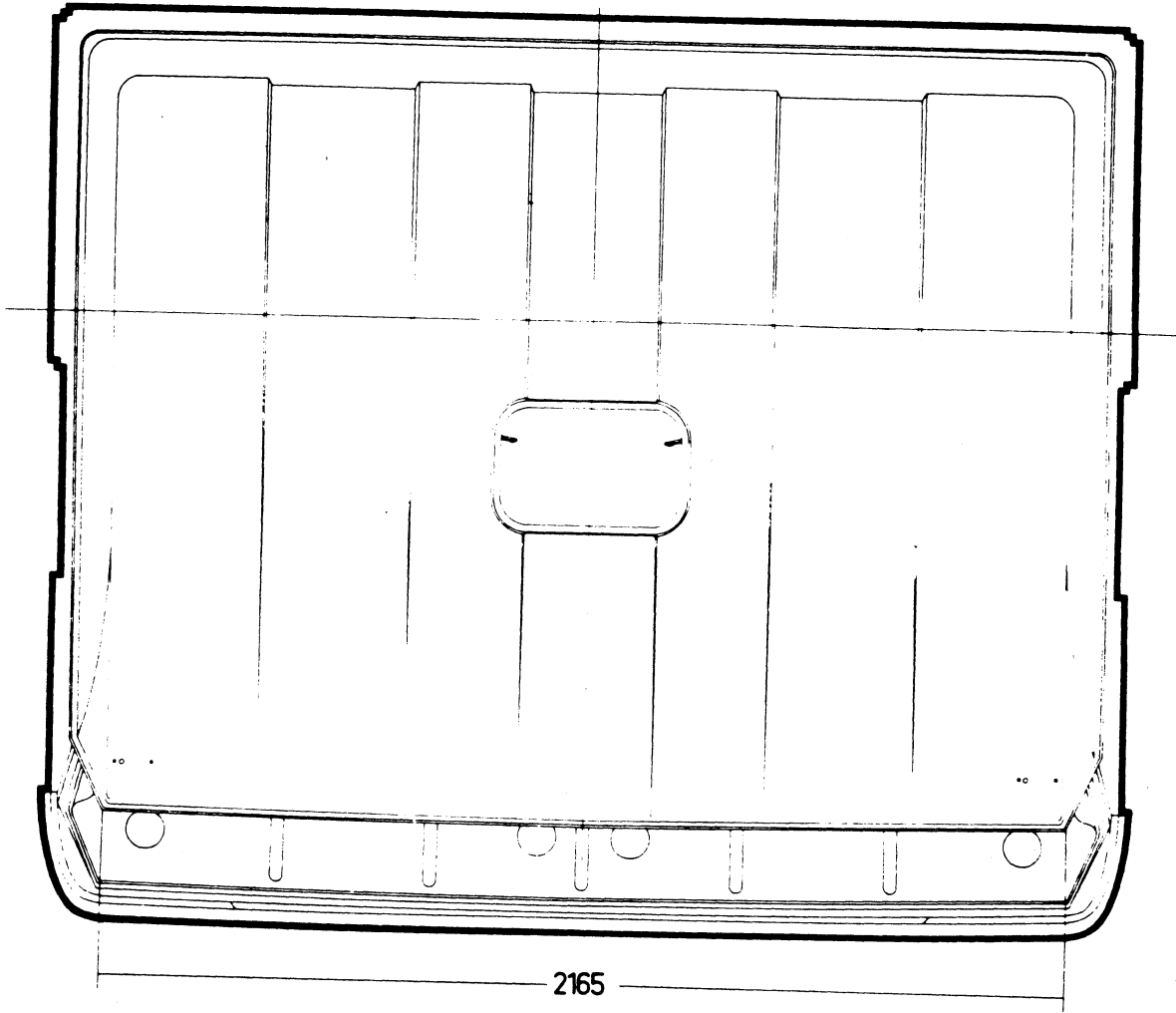
Bovenaanzicht dak kabine, lang
