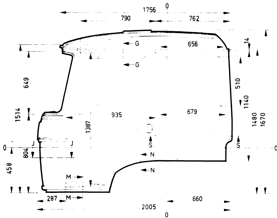
Zijaanzicht kabine, lang
