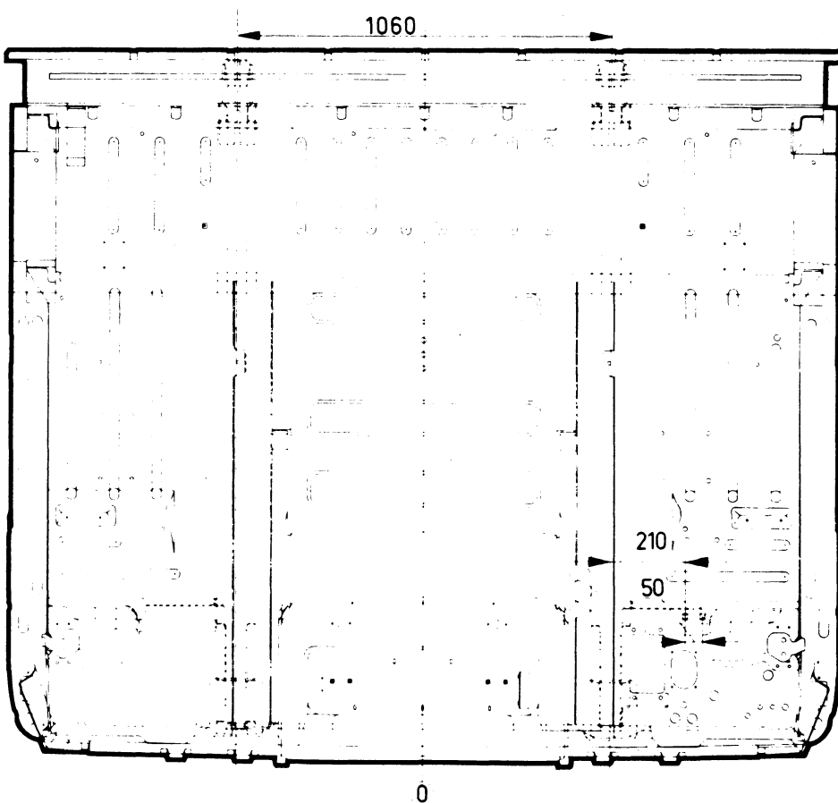
Bovenaanzicht vloer kabine, kort
