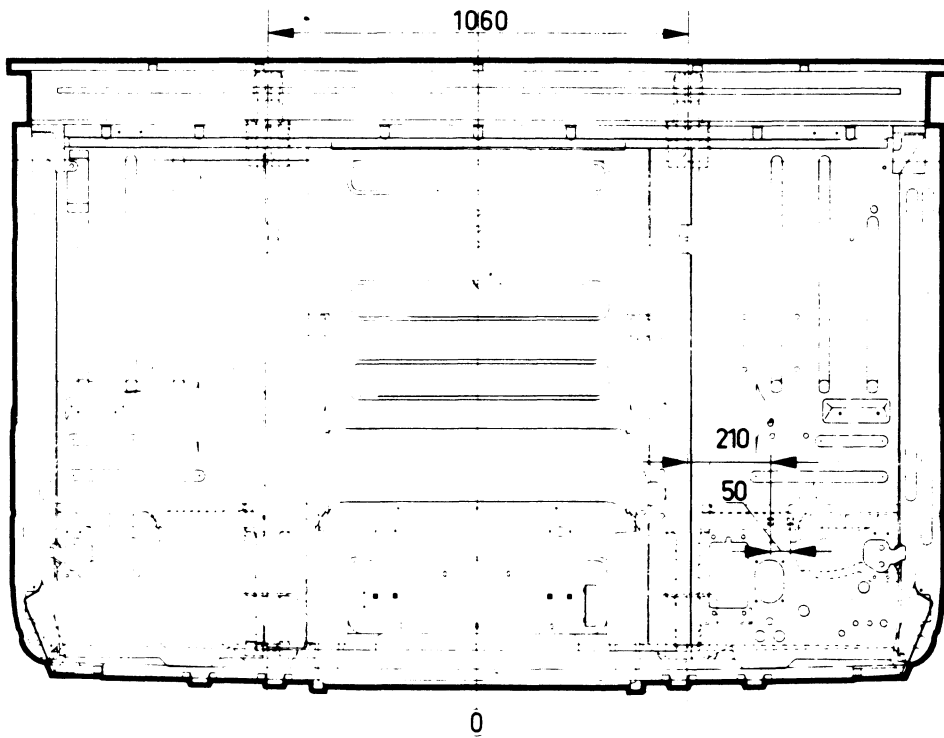
Bovenaanzicht vloer kabine, kort
