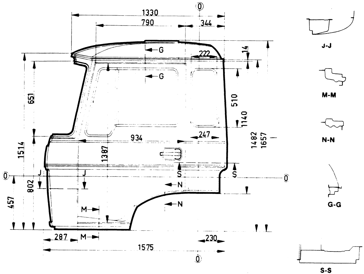
Zijaanzicht kabine, kort
