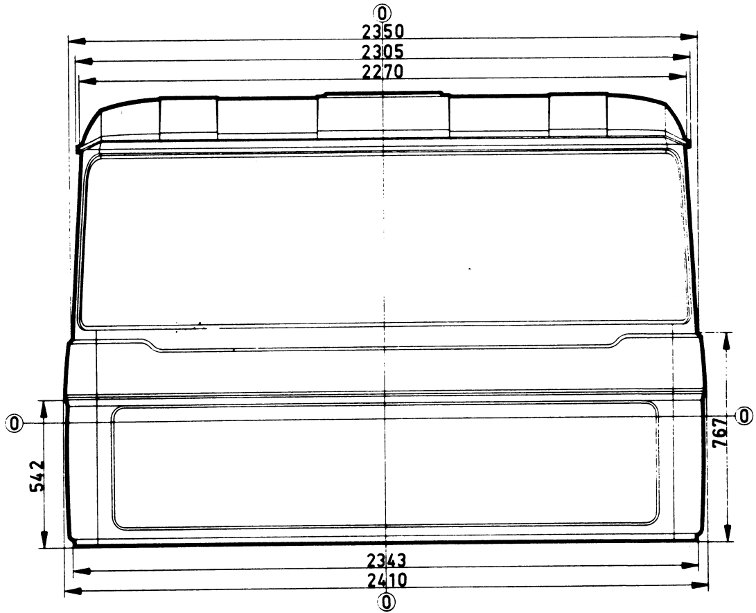
Vooranzicht kabine, lang en kort
