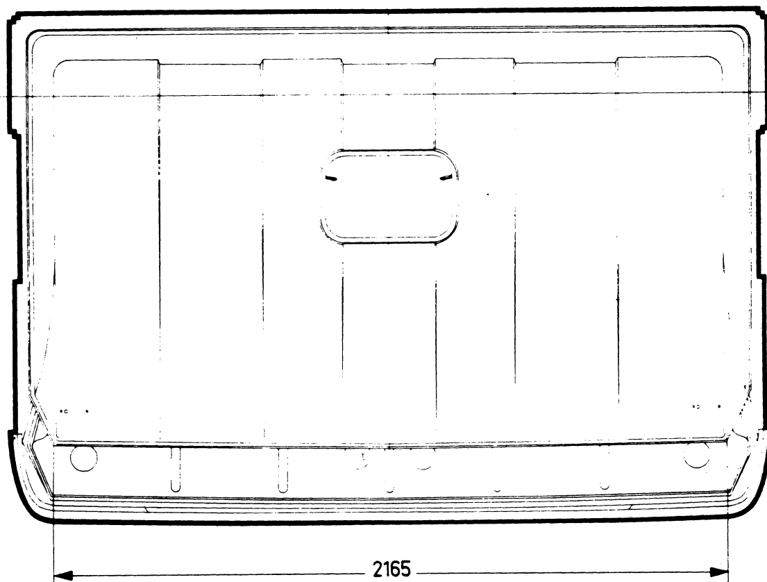
Bovenaanzicht dak kabine, kort
