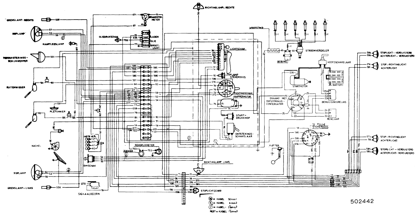
Afb. 35 Schema elektrische installatie V1600
