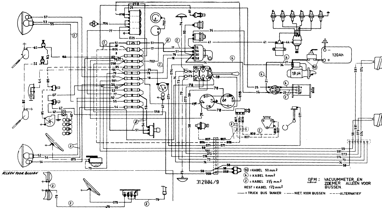
Afb. 31 Schema elektrische installatie 1100 BA 1300 BA 1600 BB en B 1600 BB
