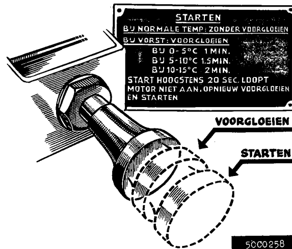
Fig. 78. De standen van het voorgloeien en starten.
