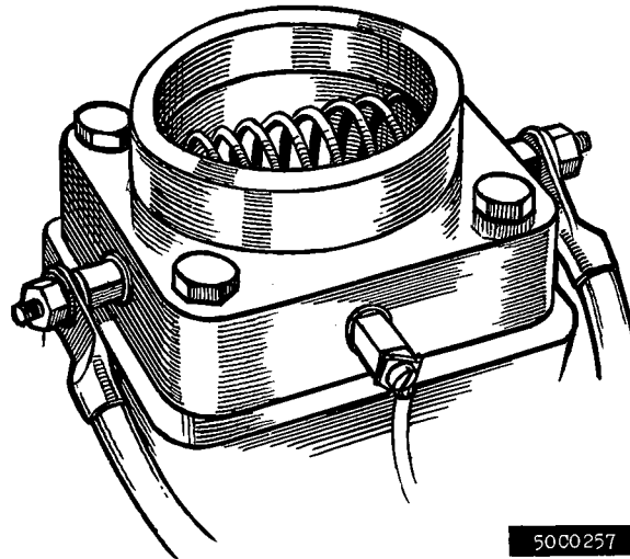
Fig. 77. De gloeispiraal gemonteerd op het inlaatspruitstuk.
