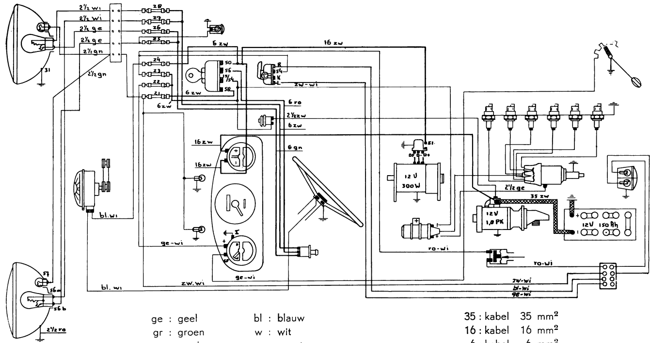
Schema elektrische installatie buschassis met benzine motor
