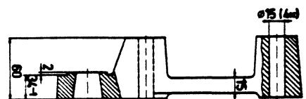
steun, hulpcilinder
