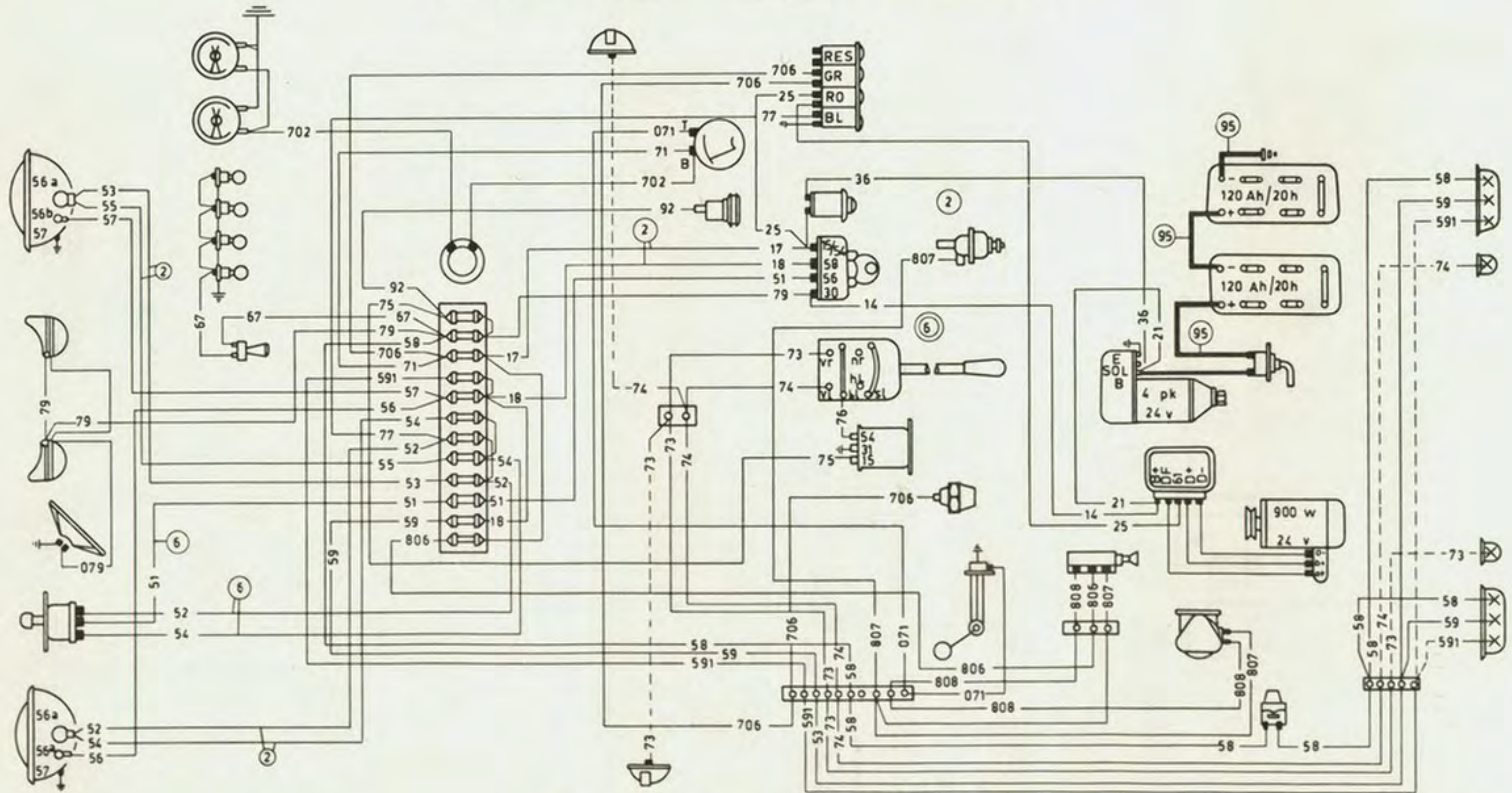
Afb. 44. Electrisch schema TB 160
