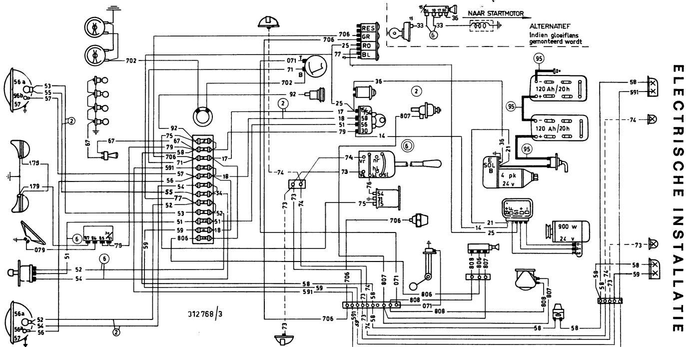
Afb. 38 Electrisch schema
