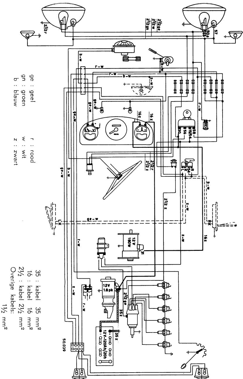
Schema elektrische installatie van vrachtautochassis met benzinemotor
