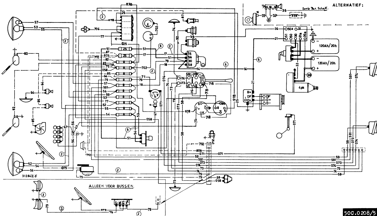
Afb. 45 Schema elektrische installatie T 1800 DS en 1900 DD/DS
