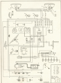
Abb. 1. Schema elektrische installatie.
